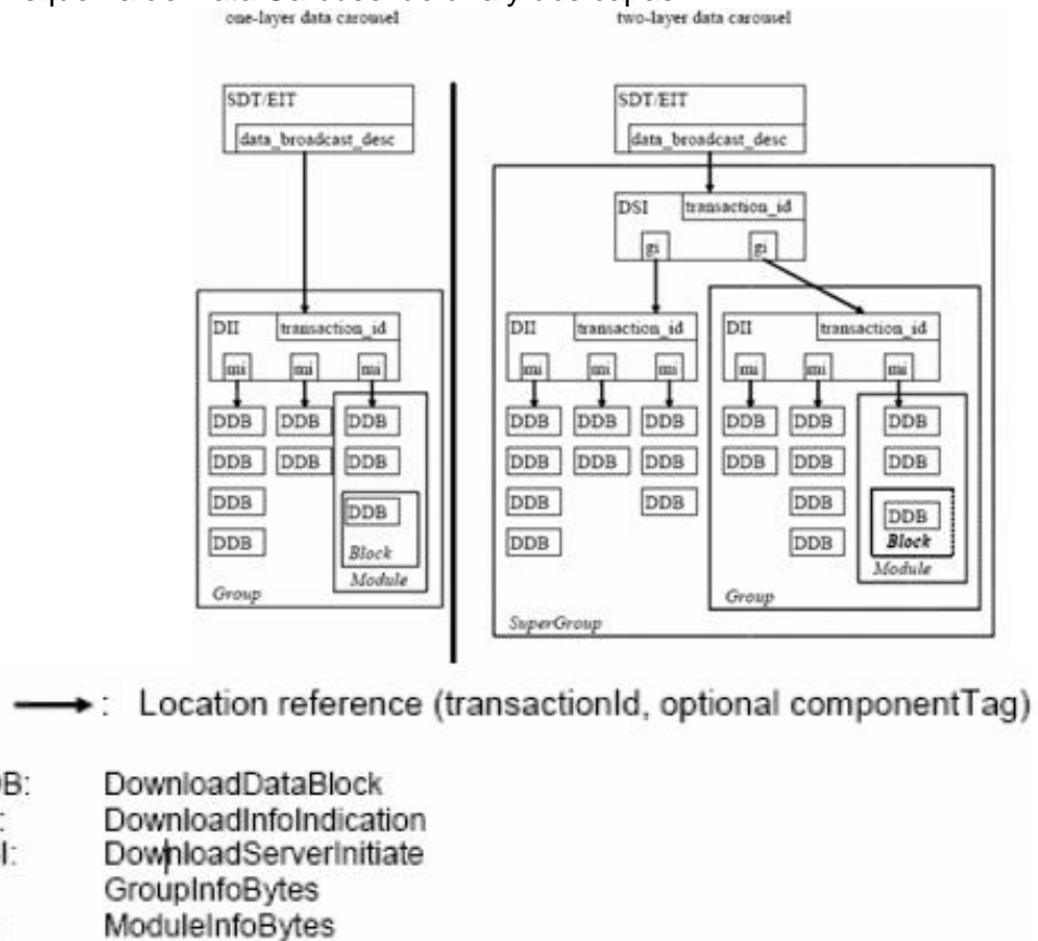
Figura 50. Esquema de Data Carousel de una y dos capas.
