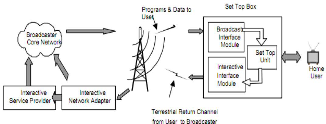
Figura 46. Red DVB-RCT.
