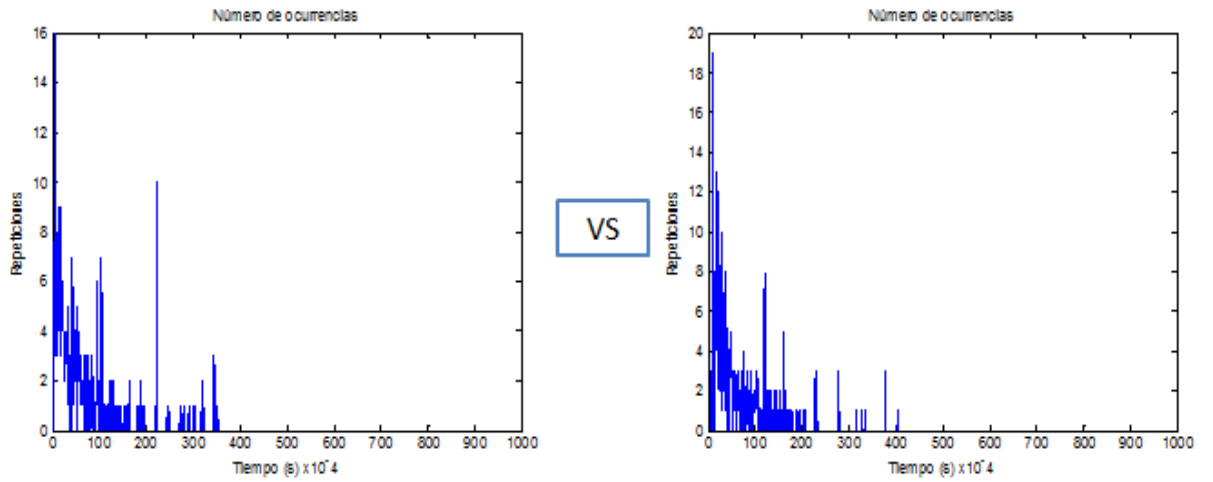
Figura 98. BW de 1Mhz Vs BW de 450Khz del nodo 2 al nodo 0.
