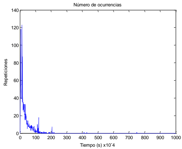
Figura 73. Número de ocurrencias del nodo 3 al nodo 0.
