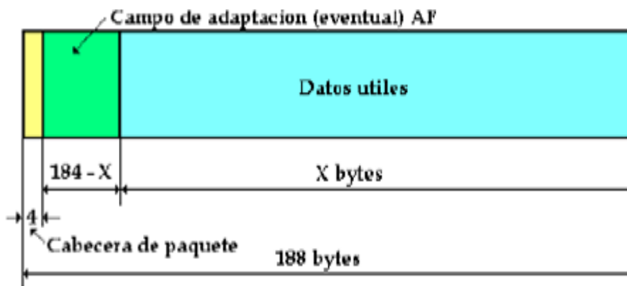
Figura 15. Construcción de un paquete de transporte.
