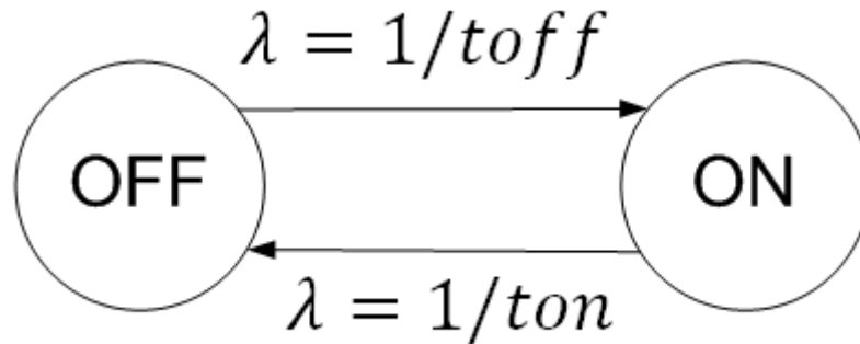
Figura 84. Modelo de fuente ON-OFF.
