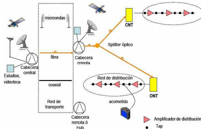
Figura 38. Red de distribución de televisión a través de cable.
