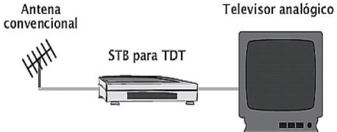
Figura 8. Recepción de TDT para un televisor analógico.
