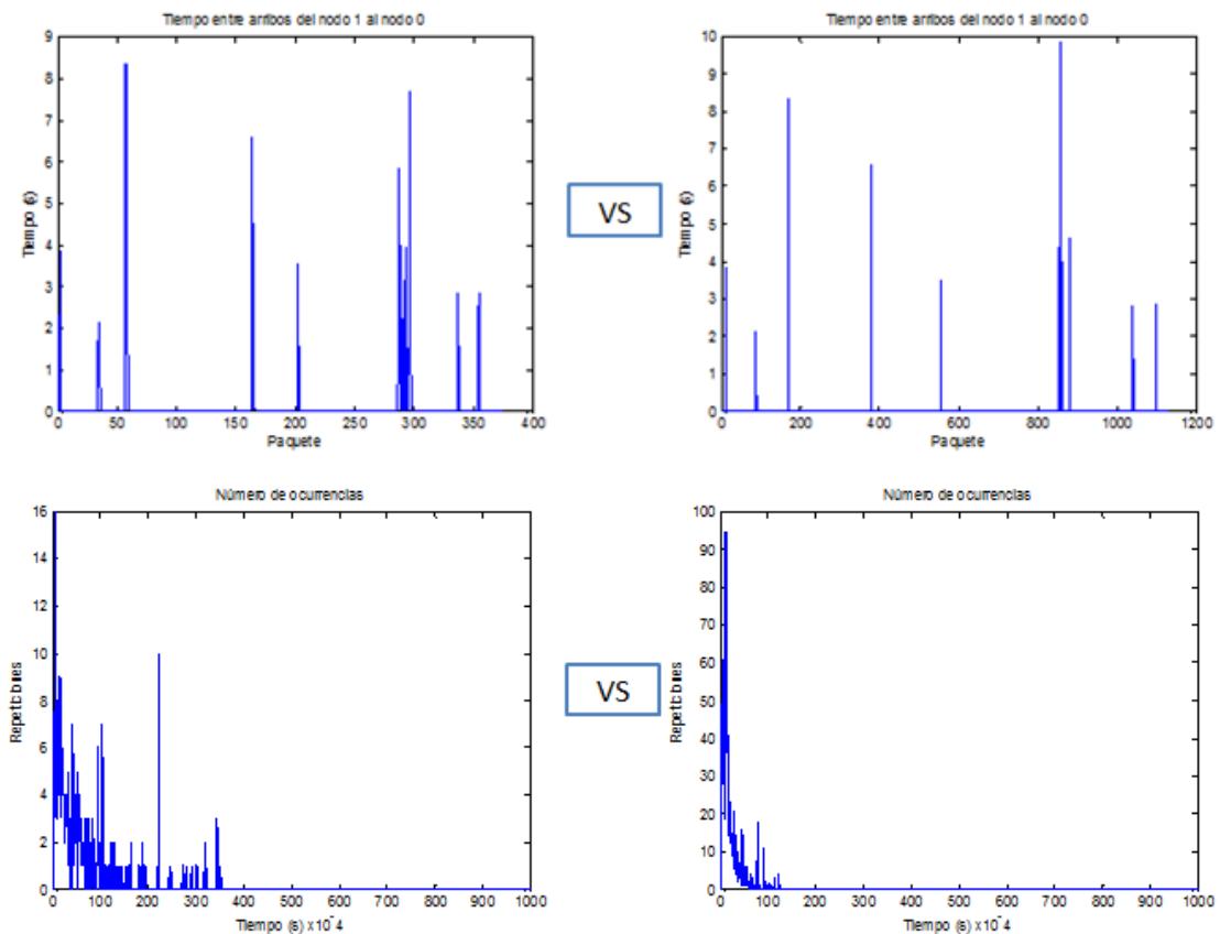
Figura 103. Velocidad de tx de 38Kbps Vs 120Kbps del nodo 1 al nodo 0.
