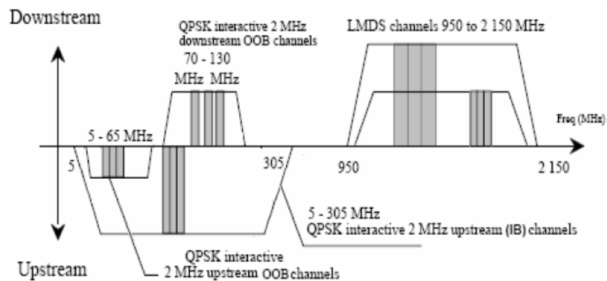
Figura 42. Rango de frecuencias para un sistema interactivo LMDS.
