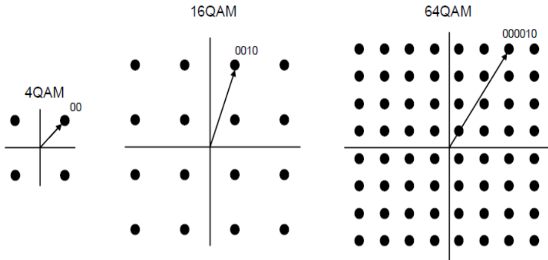
Figura 10. Constelaciones usadas en DVB-T.
