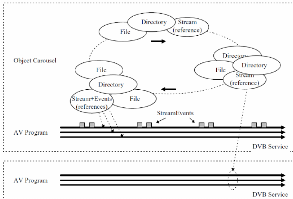
Figura 52. Esquema de como se referencian los Object Carousel en DVB.
