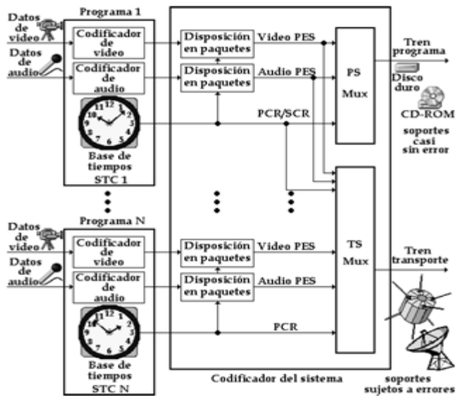
Figura 13. Esquema conceptual de la generación de transporte en MPEG-2.
