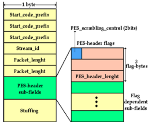
Figura 12. Cabecera de un PES en MPEG-2.
