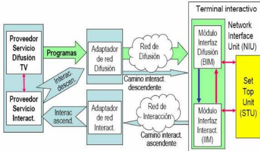
Figura 45. Modelo de referencia para interactividad en sistemas terrestres.
