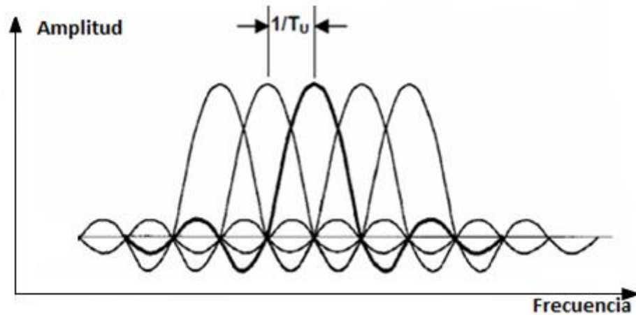
Figura 5. Ortogonalidad de subportadoras en OFDM.
