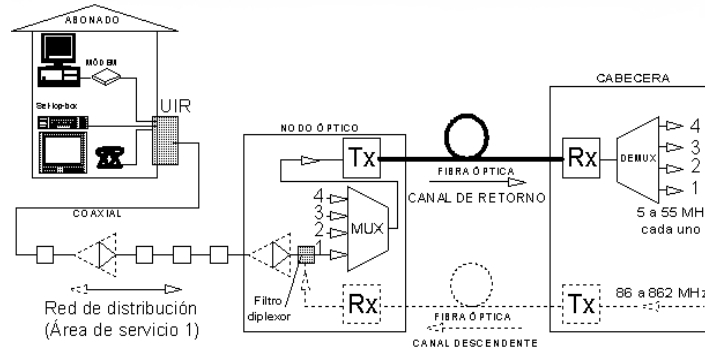
Figura 43. Canal de retorno por ADSL.
