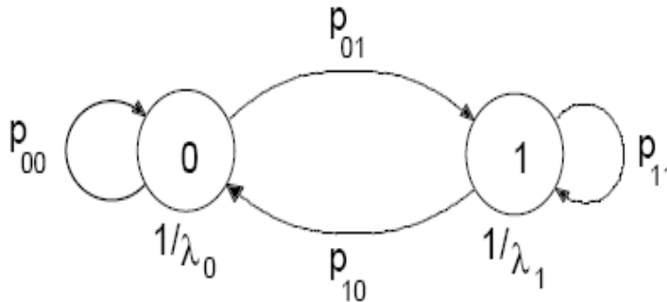
Figura 28. Cadena de Markov de dos estados.
