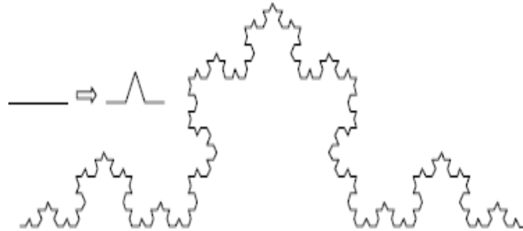
Figura 29. Copo de Nieve de Von Koch con dimensión fractal.
