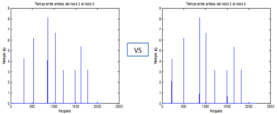
Figura 94. Latencia 100ms Vs Latencia 50ms del nodo 3 al nodo 0.
