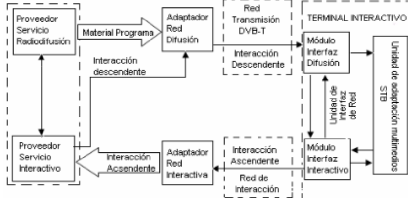
Figura 47. Diagrama de la red DVB-RCT.
