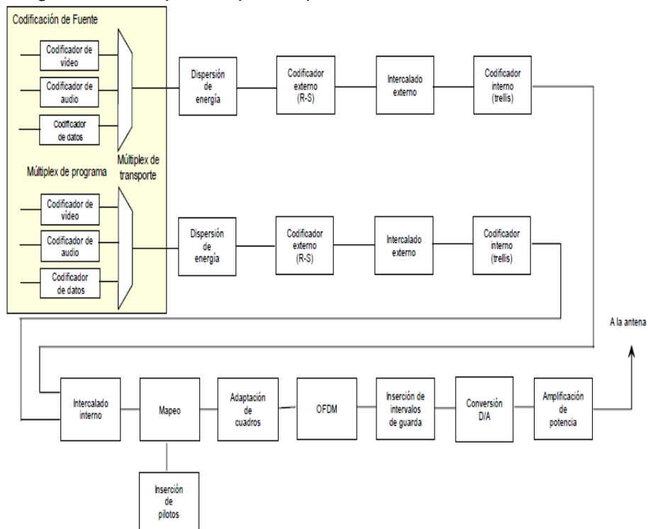
Figura 11. Diagrama de bloques empleado para el sistema DVB-T.
