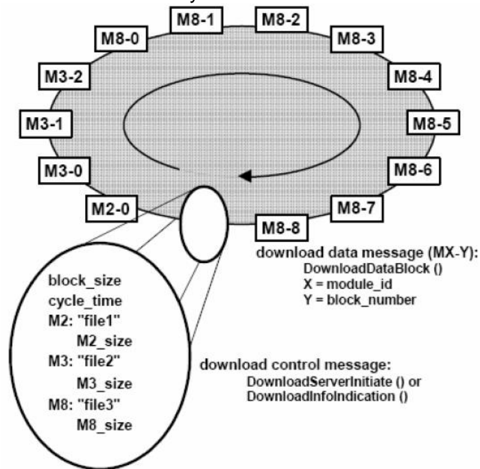
Figura 51. Esquema del Data Carousel y sus Módulos.
