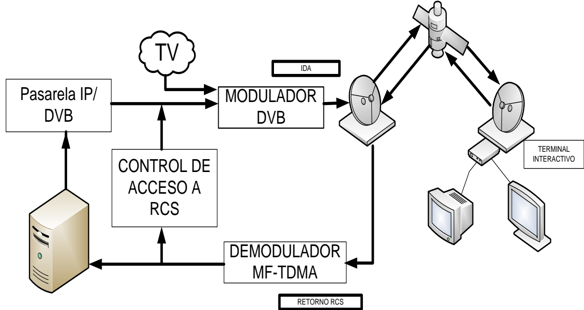
Figura 35. Red satelital bidireccional.
