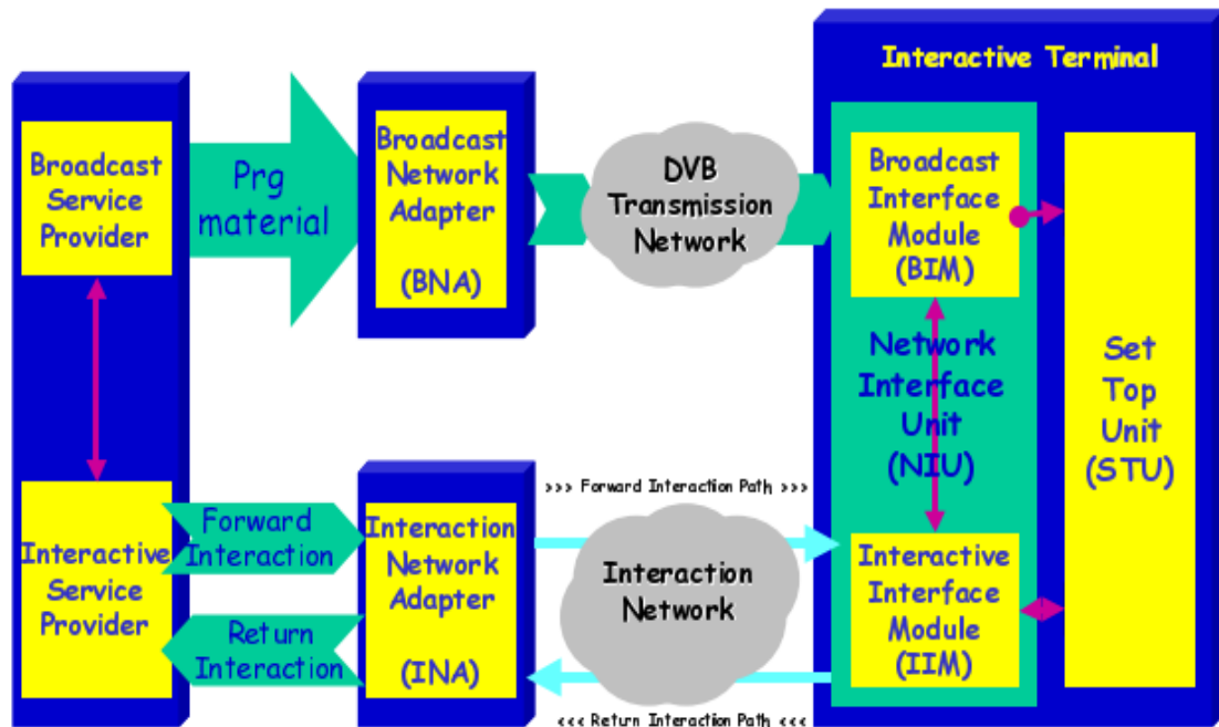
Figura 44. Sistema genérico de modelo de referencia para interactividad.
