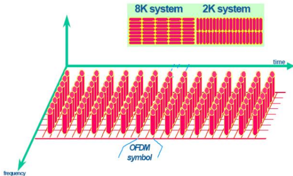
Figura 6. Transmisión de símbolos OFDM en dominio de frecuencia y tiempo.
